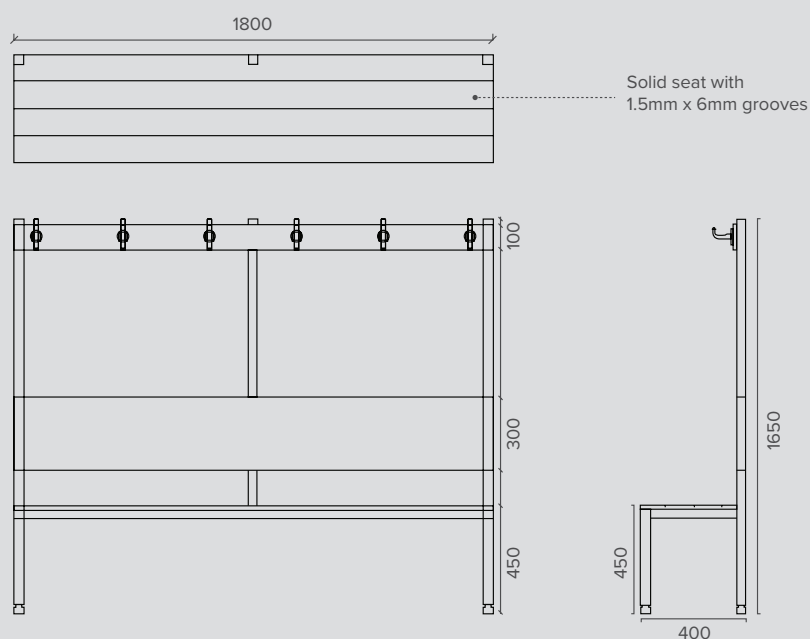
Hook Type 2116
