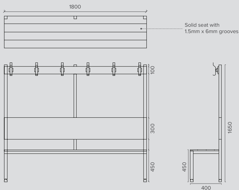
Hook Type 76827
