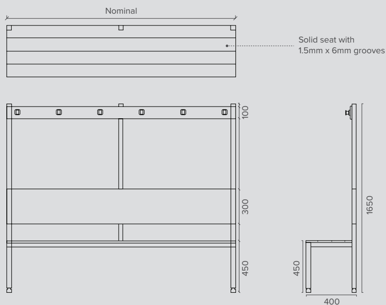
Hook Type 76717
